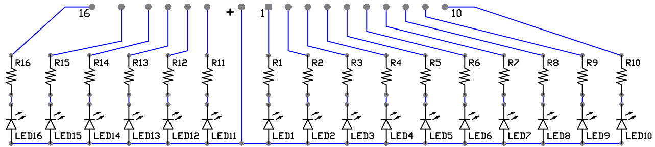
PCB-DSPB16-1
