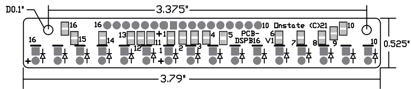
PCB-DSPB16-1
