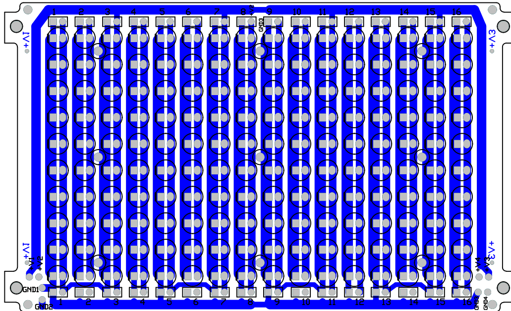
IA160 Bottom Layer Trace
