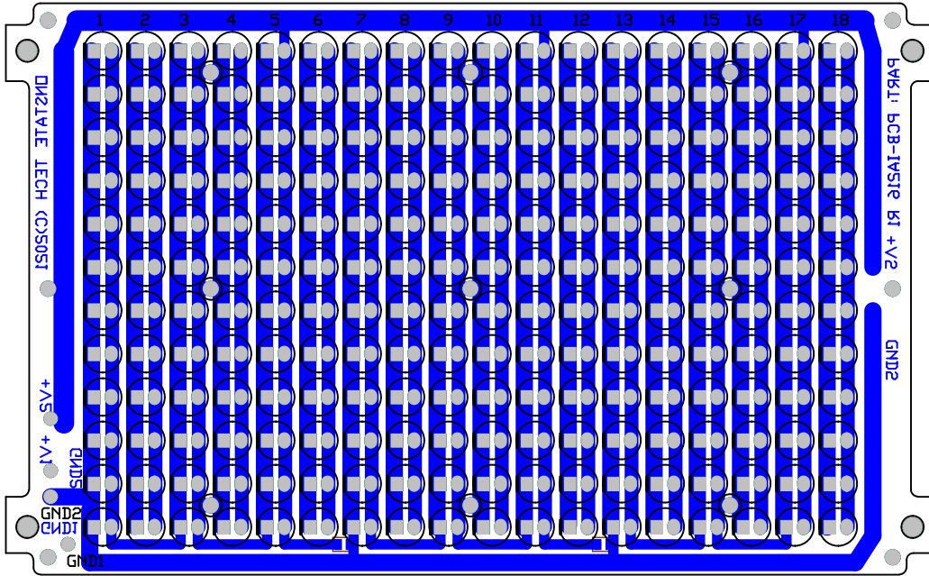
BOTTOM LAYER TRACES
