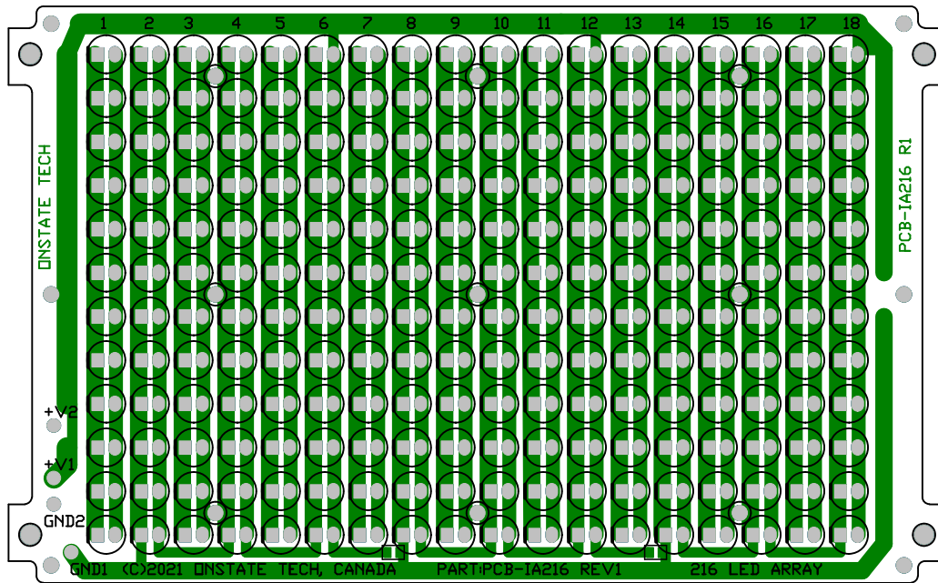
TOP LAYER TRACES
