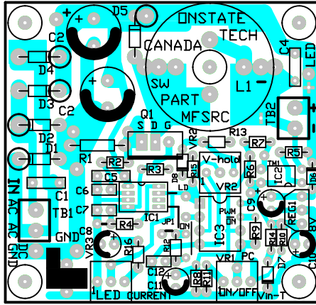
BOTTOM LAYER
