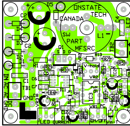
TOP LAYER
